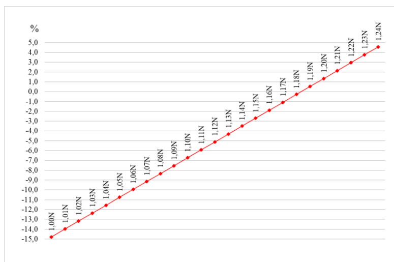
График 3. Предел повышения расчетных нагрузок стандартной несущей способности сваи
