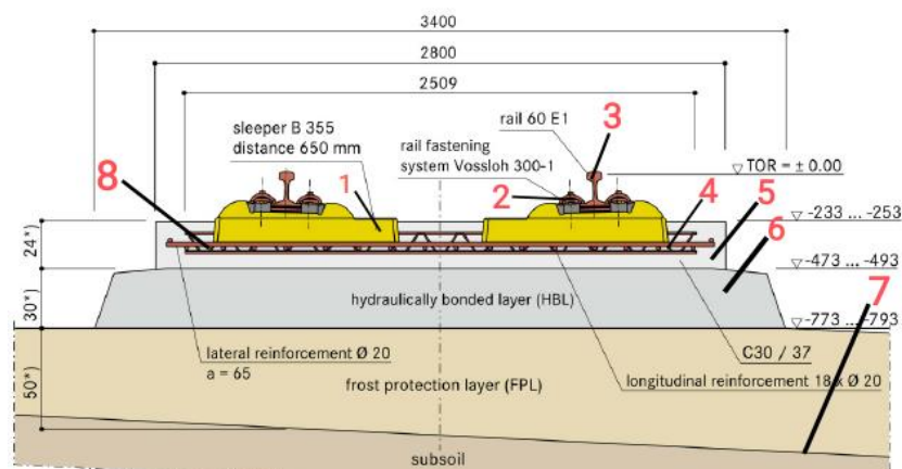
3-rasm. RHEDA tipidagi ballastsiz relsosti asosi:
