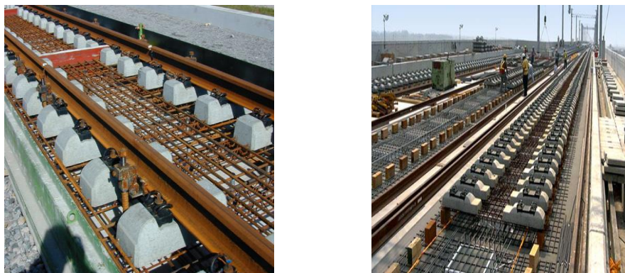
2-rasm. Ballastsiz yoʻlni betonlashga tayyorlash.
