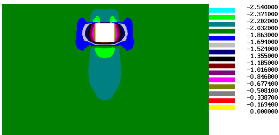
Рис.3. Распределения вертикальных главных напряжений, (МПа)
