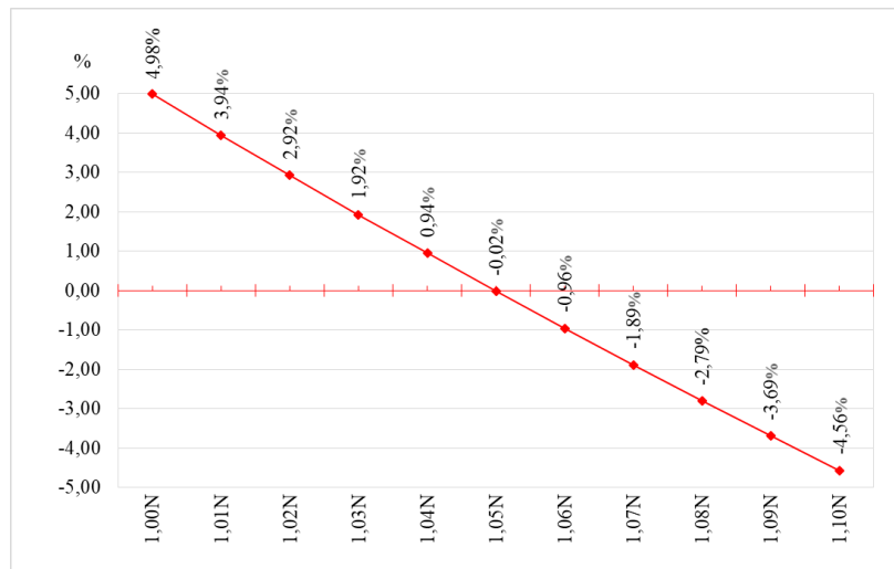
График 2. Предел повышения нагрузки на расчетную поверхность фундамента
