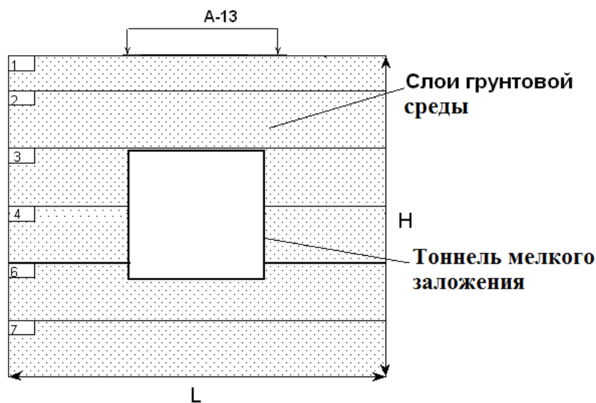
Рис.1. Расчетная схема плоской области «тоннель-грунт»,
