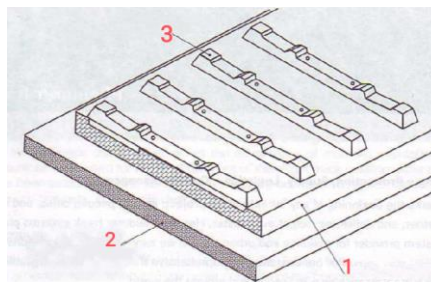
5 - rasm. Sublin tipidagi ballastsiz yo‘l konstruksiyasi.
