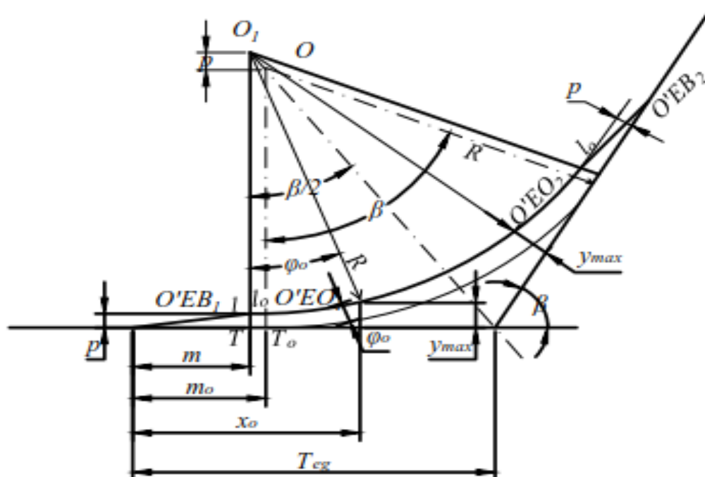
1 – rasm O‘tish egri chizig‘ini aylanma egrisini ichkariga surish (ko‘chirish) yo‘li bilan joylashtirish sxemasi.
