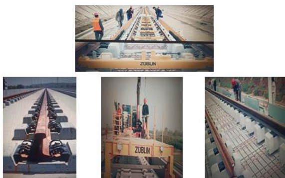
6-rasm. Sublin tipidagi yo‘l konstruksiyasi qurilish jarayoni.
