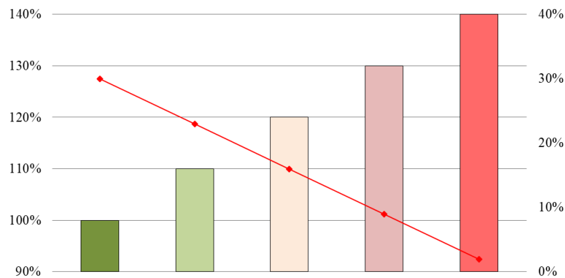
График 1. Динамика влияния увеличения расчетных нагрузок на несущую способность
